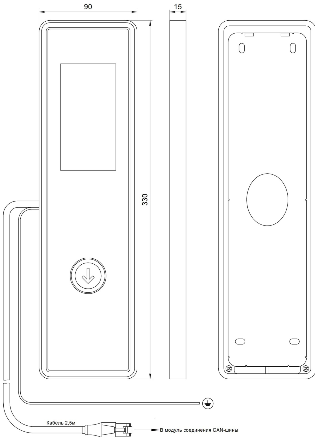
Рис.1 Внешний вид, габаритные и установочные размеры Вызывного поста ОБСИДИАН (жгут RJ45) НШЕК.468381.220-01
